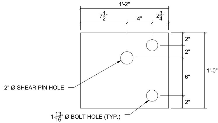
SSP-2 t = \frac{5}{8} ", A572-50, QTY: 2
