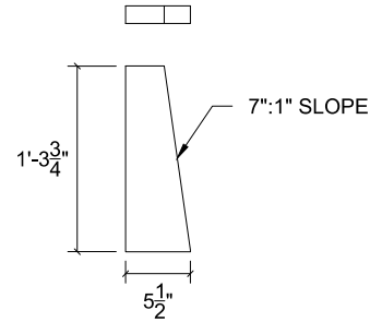
4D: 2x6 QTY: 8
