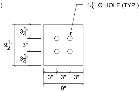
PLATE E t = 1", A572-50, QTY: 4
