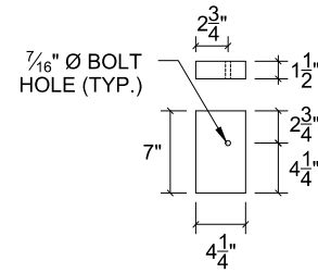
1G: 2x6 QTY: 2
