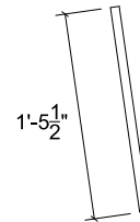
4C: 2x6 QTY: 2
