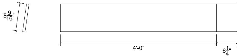
SIDE PLYWOOD: 1P, 1Q QTY: 2
