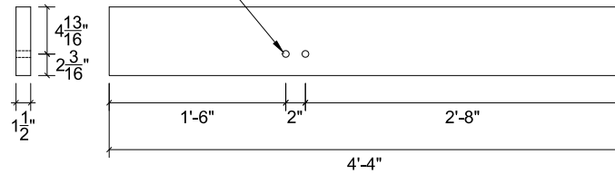
1D: 2x8 QTY: 4
