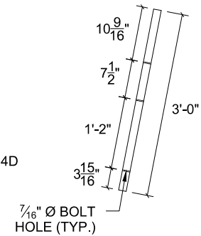
2X4 TIMBER 4E
