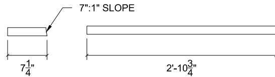
4A: 2x8 QTY: 2
