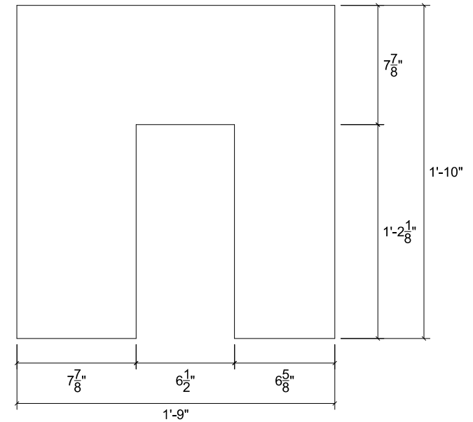
SAP-2 t = 1", A572-50, QTY: 1
