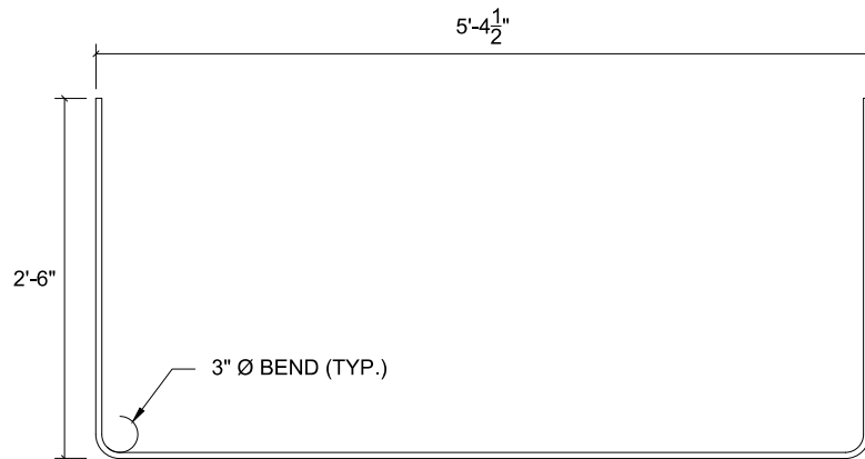
BAR 4B BAR SIZE: #4, QTY:8
