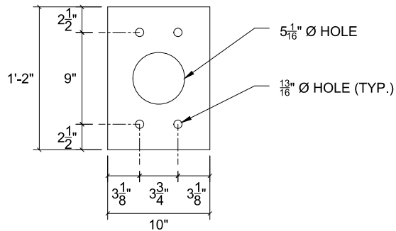
AP2 t = 1/2", ALUMINUM 6061 T6, QTY:2
