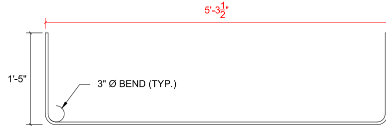
BAR 4A BAR SIZE: #4, QTY:12
