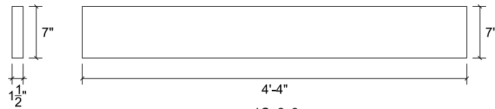
1C: 2x8 QTY: 7
