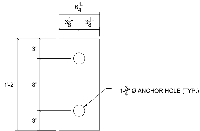
SAP-1 t = 1", A572-50, QTY: 4
