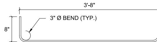
BAR 4C BAR SIZE: #4, QTY:4
