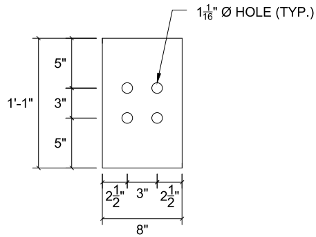
PLATE D t = 1", A572-50, QTY: 4
