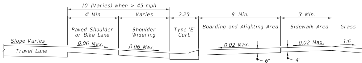
SECTION A-A
