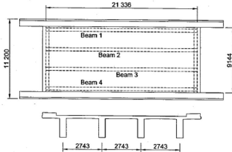
Figure 38—Sainte-Emelie-de-l'Energie bridge (Labossiere et al., 2000)
