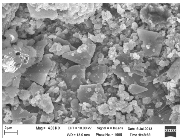
(d) 4,000X
