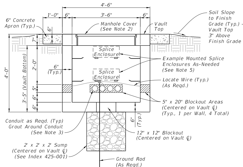
SECTION D-D
