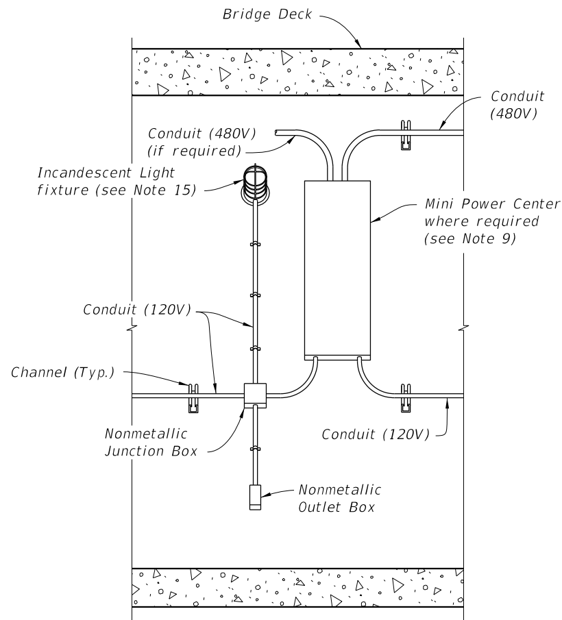
SECTION A-A
