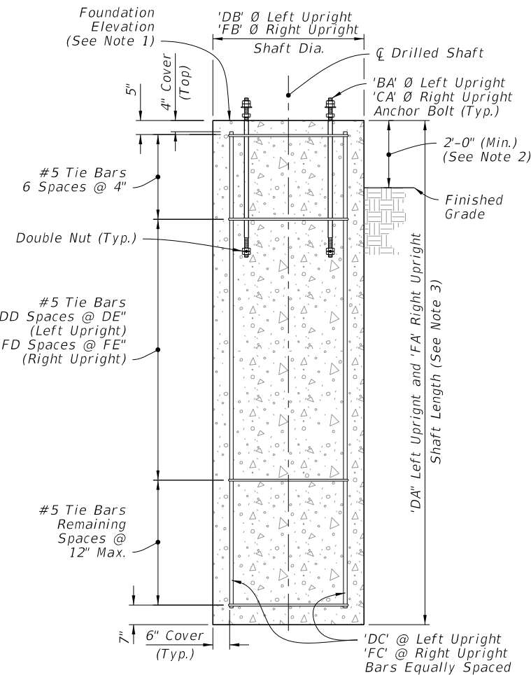
ELEVATION
