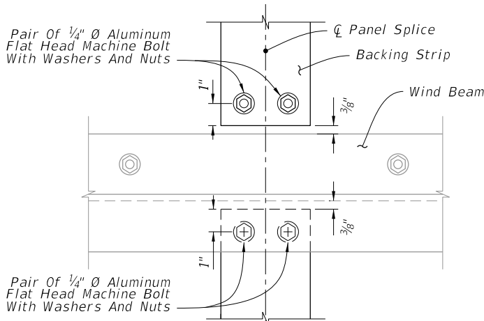
ELEVATION
