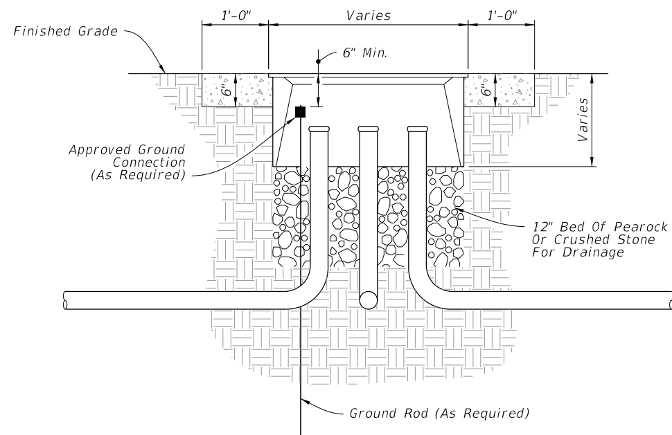
ELEVATION
