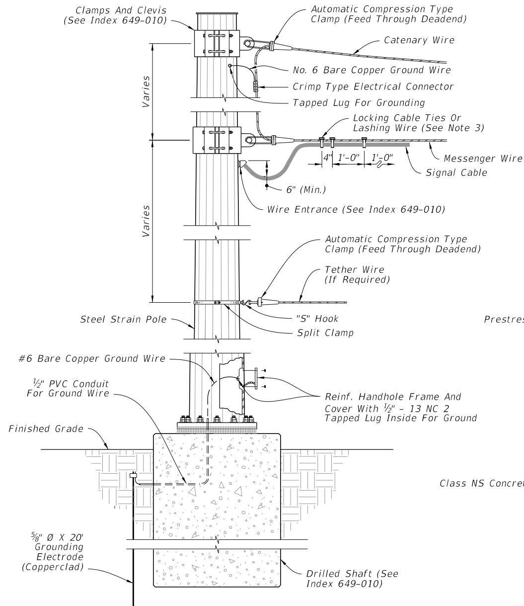
ELEVATION
