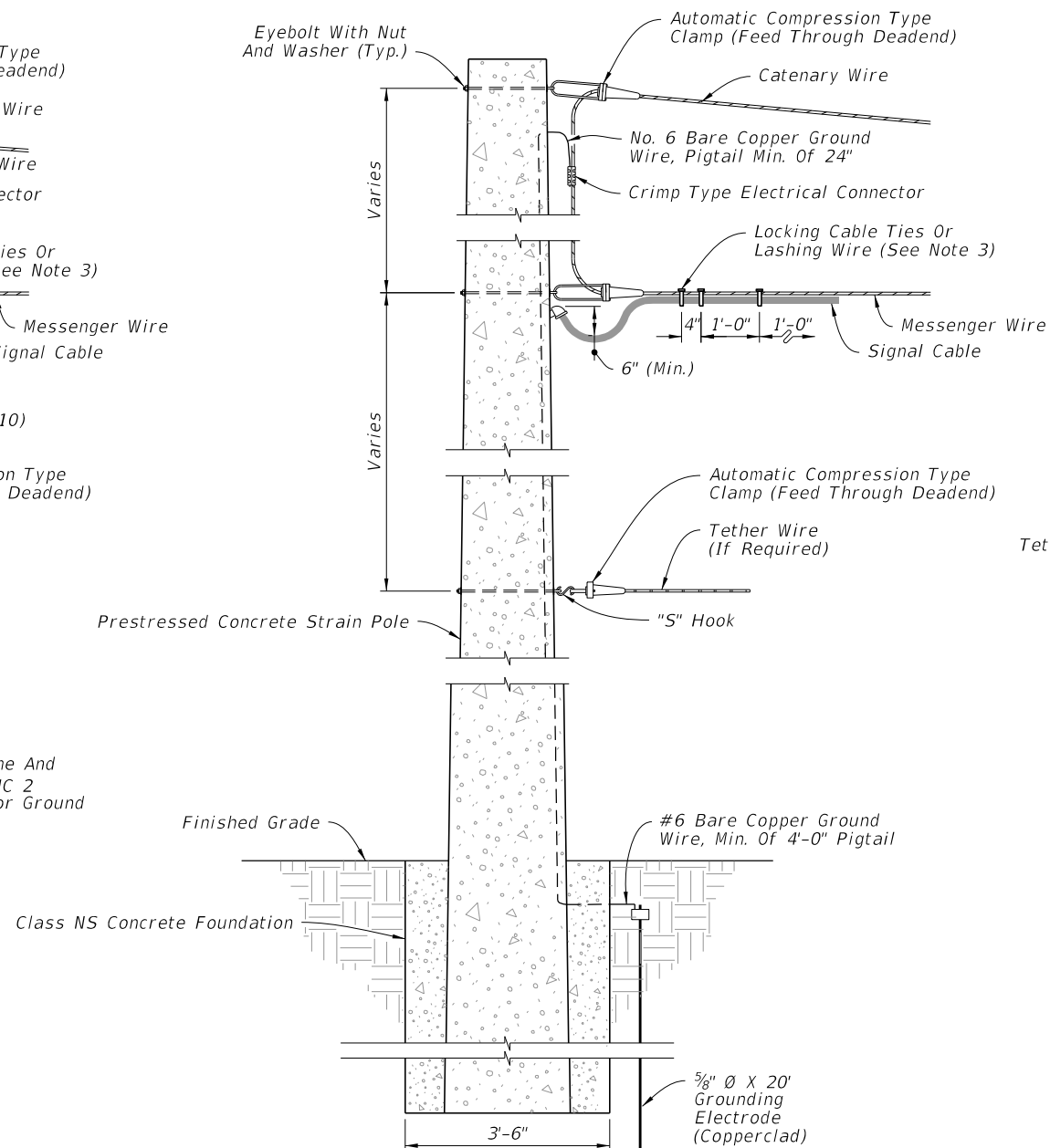
ELEVATION
