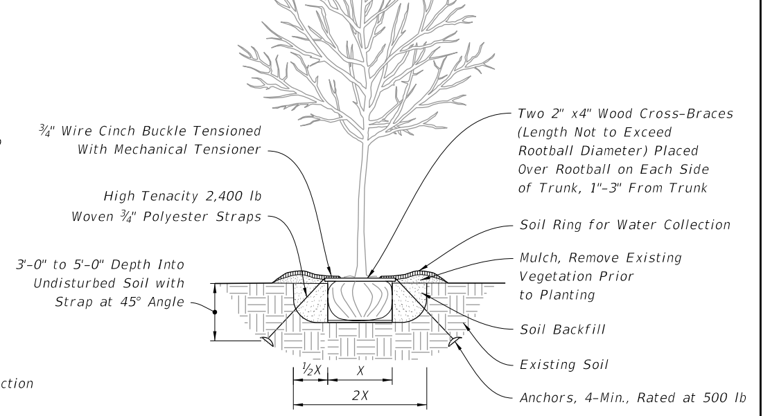
ELEVATION
