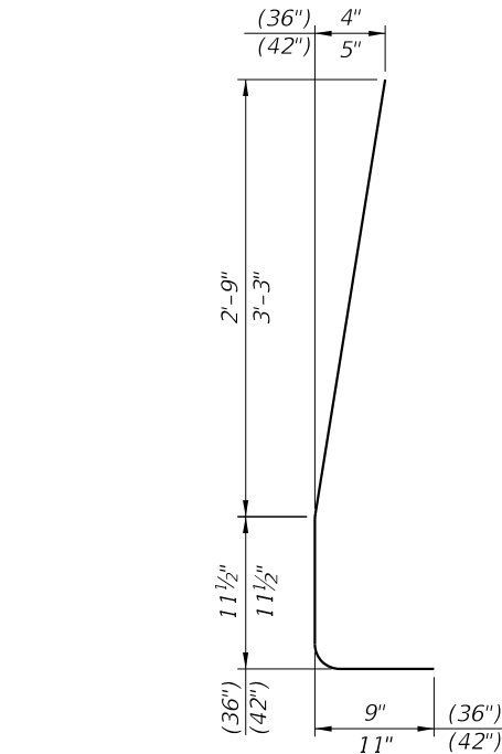
STIRRUP BAR 5V1
