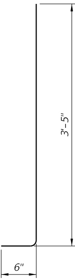
STIRRUP BAR 5V4
