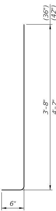
STIRRUP BAR 5V2
