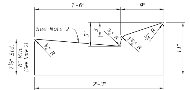
TYPE E
