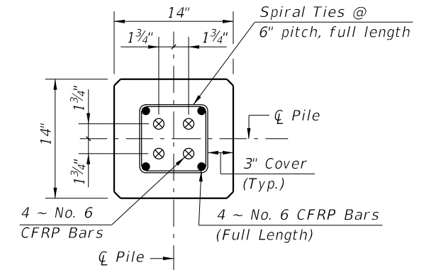
SECTION D-D
