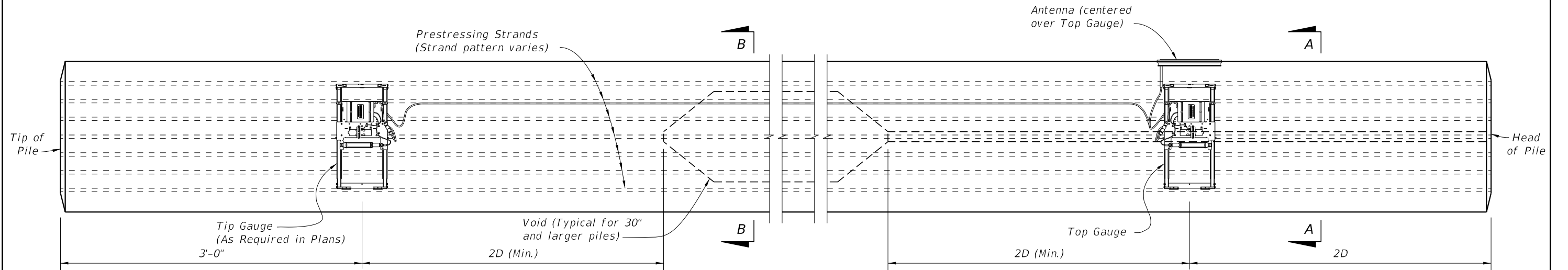
ELEVATION
