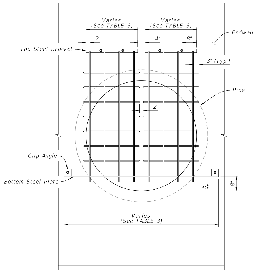
END ELEVATION
