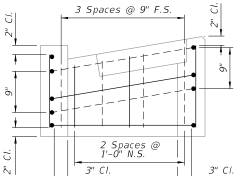
SECTION D-D
