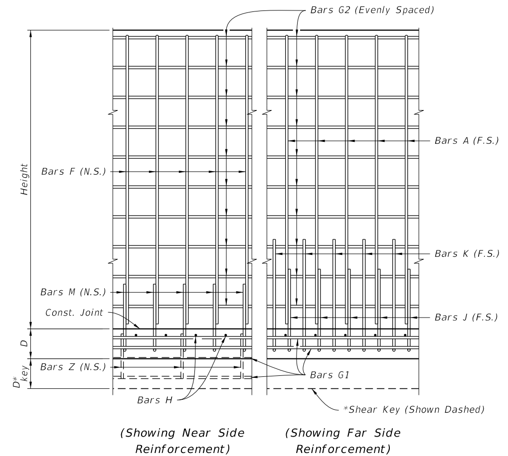
VIEW A-A
