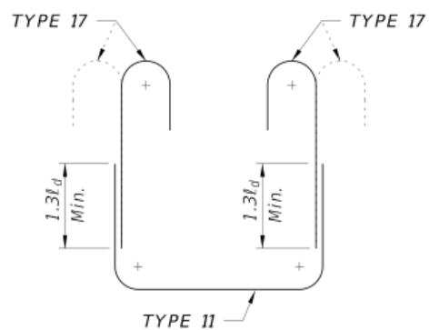
OPEN STIRRUP 3
