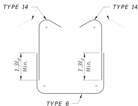
OPEN STIRRUP 2
