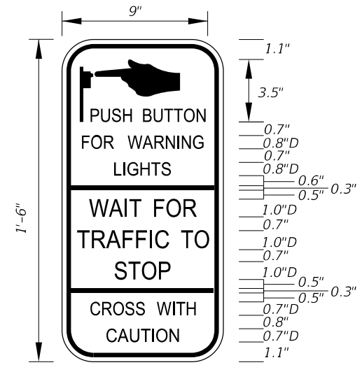
FTP-033-25 9" X 1'-6" 1.5" Radii 1/4" Border
