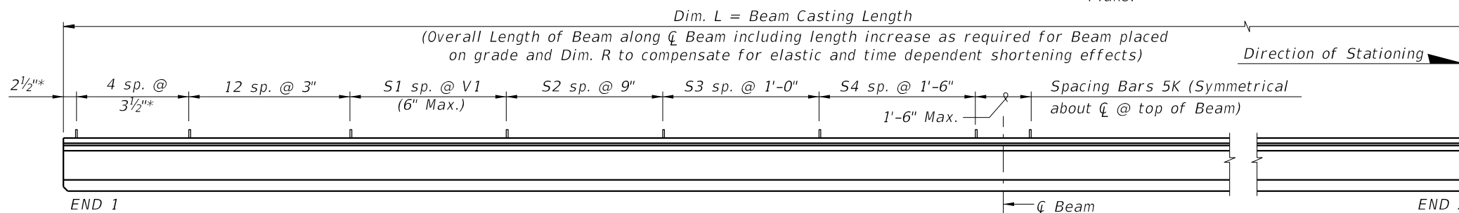
ELEVATION
