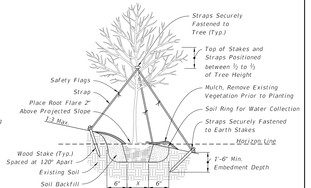
ELEVATION
