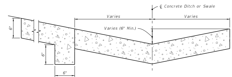
SECTION DD
