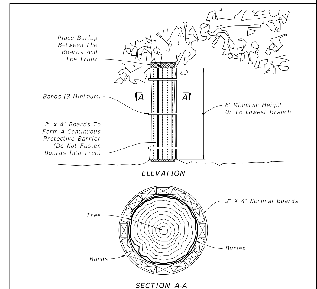
SECTION A-A
