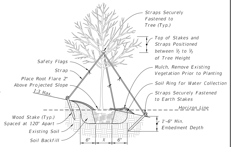
ELEVATION
