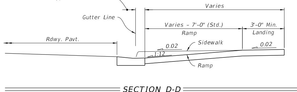
SECTION D-D
