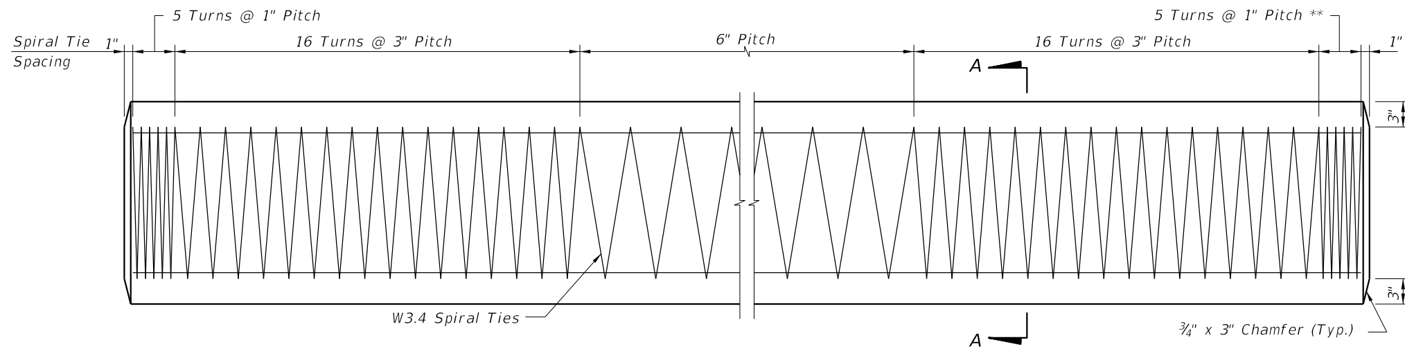
ELEVATION
