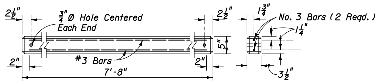
PRECAST BRACE
