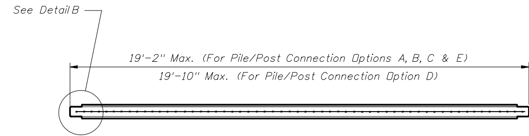
SECTION D-D
